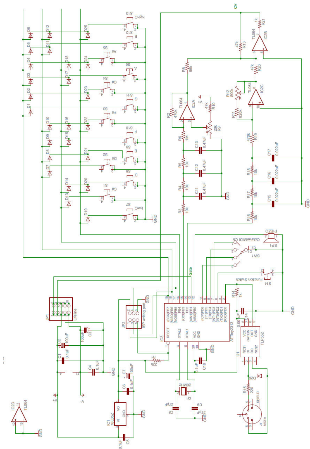
図 2-3 Mini Board II の回路図
