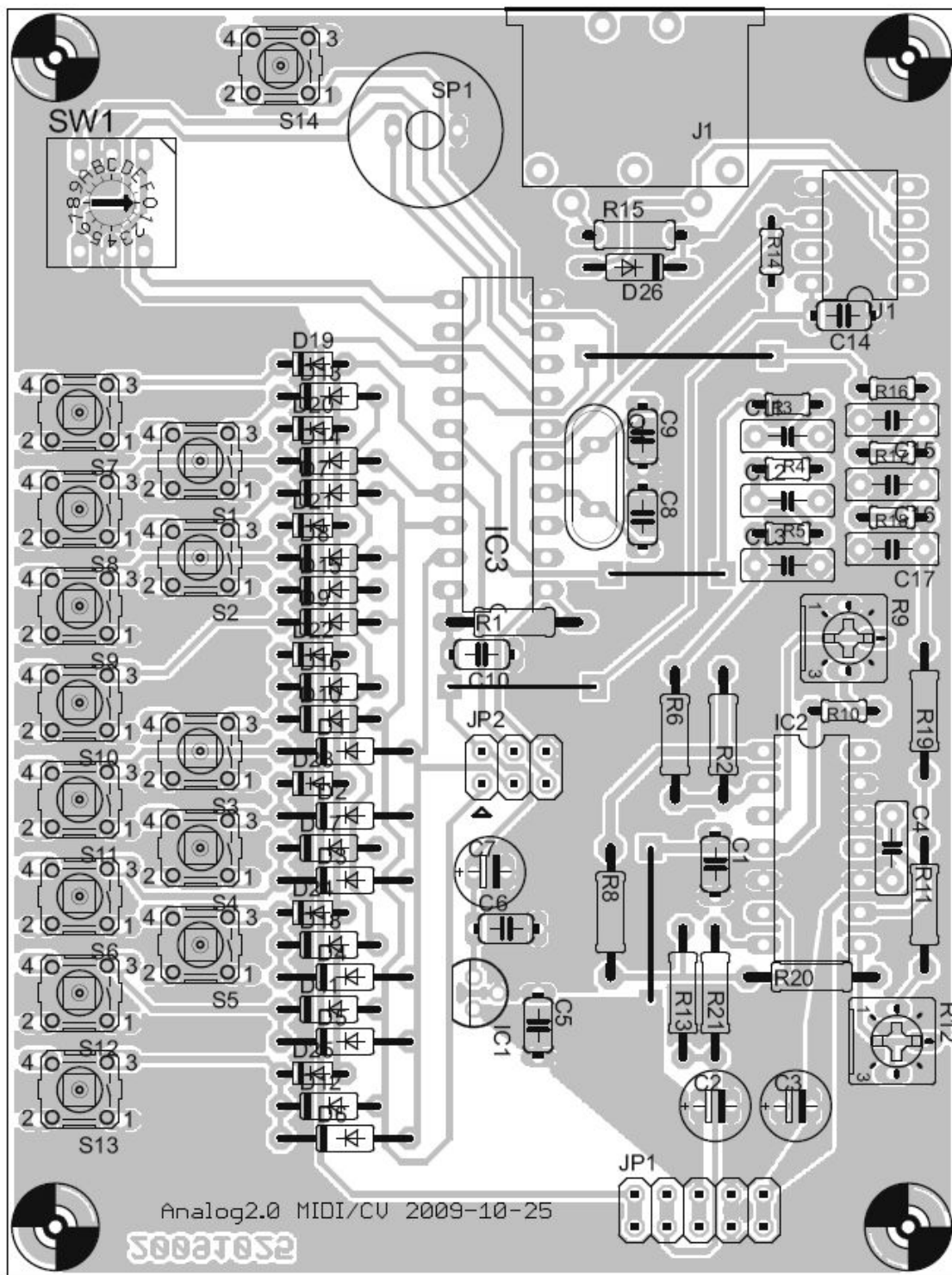
図 2-4 Mini Board 基板の配線図
