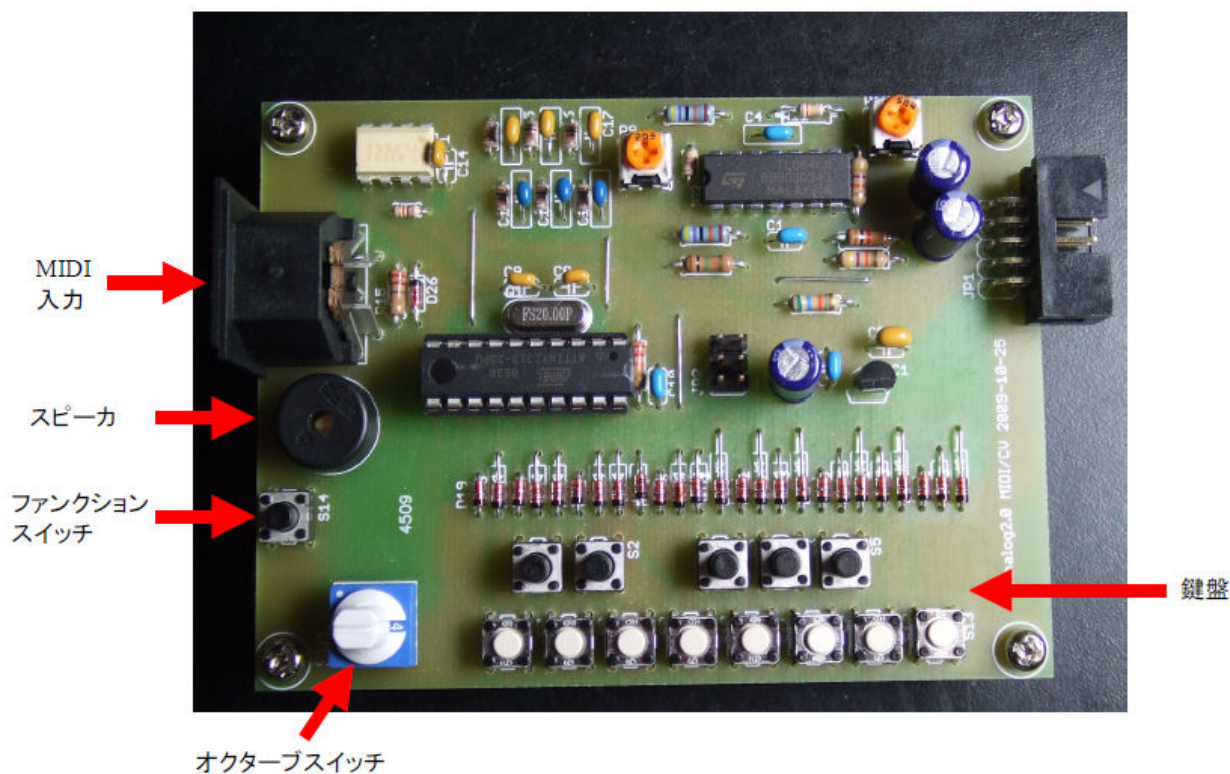
図 2-1 MInI Board II の外観
